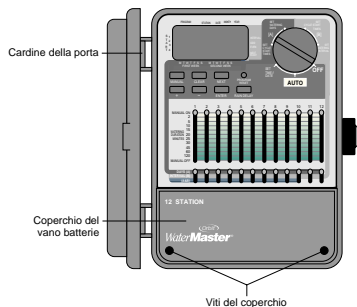
FIGURA 3: Programmatore per montaggio esterno, coperchio della morsetteria
